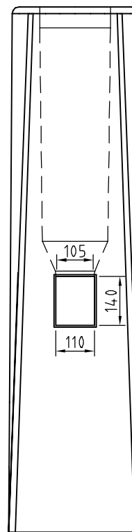
B-B 1:15
