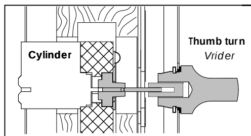
Thumb turn for the inside Vrider på indvendig side
