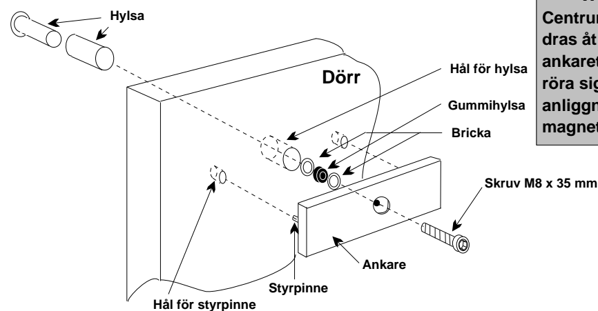
Fig 2. Utåtgående dörr med smal dörr karm Extra skruvhål kan göras i den främre delen på montage plattan. Borra 5 mm hål och försänk med 10 mm borrhål det finns 2 centrumlinjer på montageplattan som förenklar borring.
