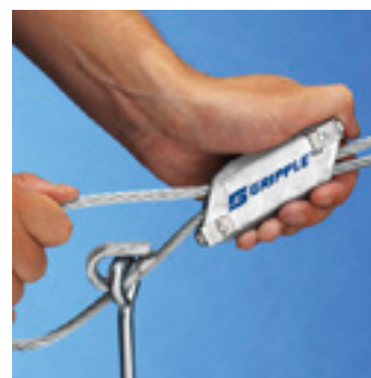
Steg 3 Tryck igenom vajern genom den fria kanalen på låset. Se till att trycka ut minst 75mm av vajer.
