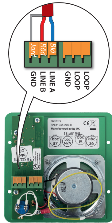
Inkoppling av SAC-SAFE-TEL C2RRG
