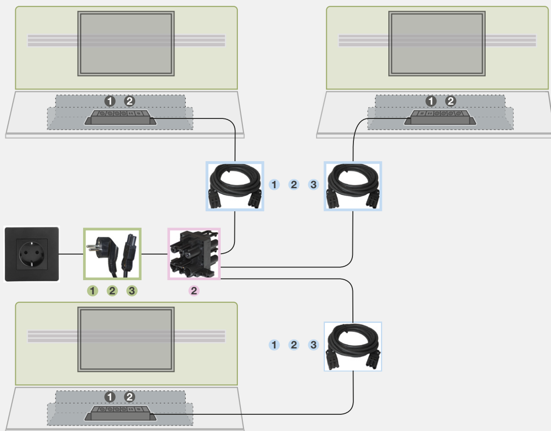
Koppling för 3 arbetsplatser, med 935-T2UD och/eller 935-T5UD
