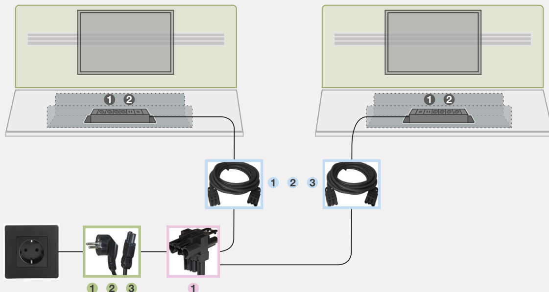
Koppling för 3 arbetsplatser, med 935-T2UD och/eller 935-T5UD
