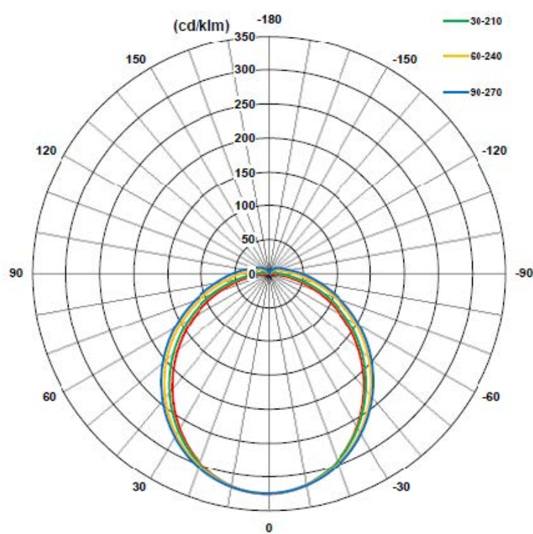
Ljusdiagram 44W Opal Kupa
