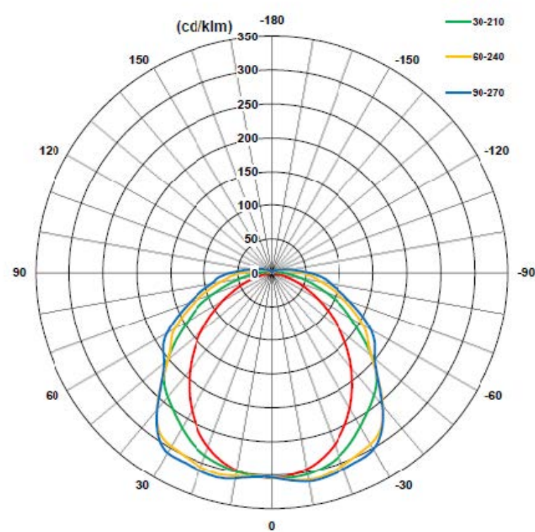
Ljusdiagram 44W Klar Kupa
