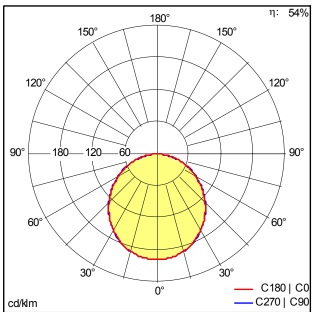
Slim_DL_4inch_8W.ltd
